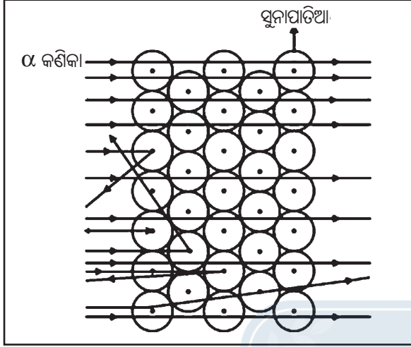
ଚିତ୍ର 4.2 ରଦରଫୋର୍ଡଙ୍କ ସୁନାପାତିଆ ପରୀକ୍ଷା
