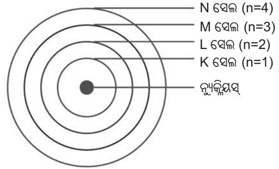
ଚିତ୍ର 4.3 ପରମାଣୁର କେତୋଟି ଶକ୍ତିସ୍ତର
