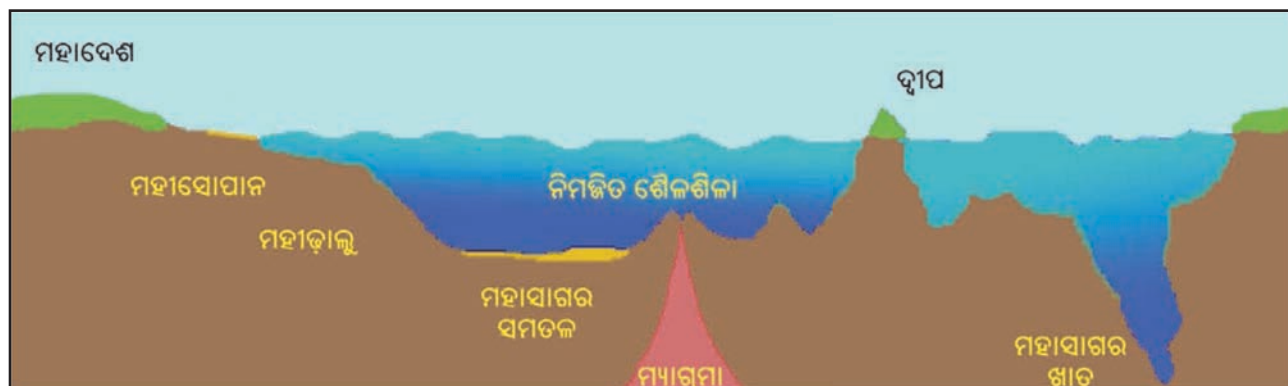
ଚିତ୍ର. ୩.୫: ମହାସୋପାନ, ମହାଭାଲୁ, ସାଗର ତଳ, ମହାସାଗର ଖାତ ଓ ନିମଜ୍ଜିତ ଶୈଳଶିଳା
